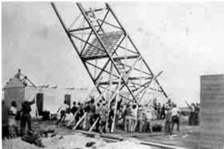
Aufrichtung des vormontierten Wach- und Wasserturms. Foto: Hans Bloch, Shavei Zion
